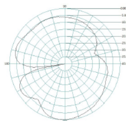
E-PLANE
